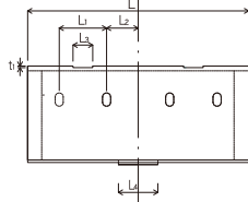
断面図(φ100,φ150)
