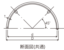
断面図(共通)
